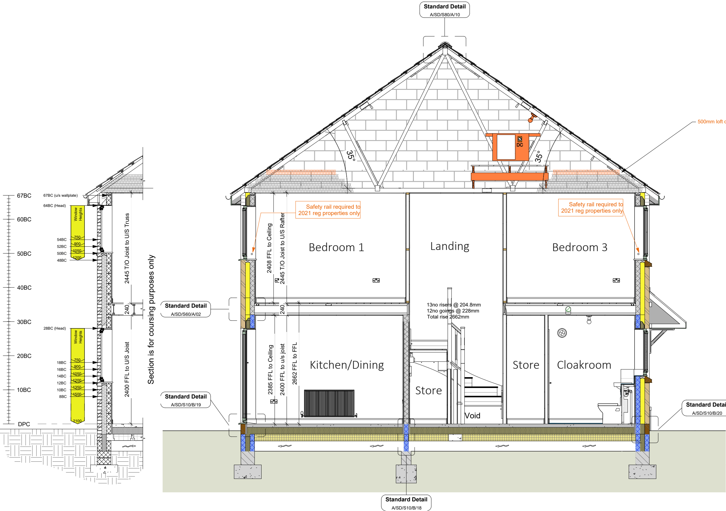
B Section B - B 1 : 50
